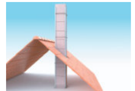
Standsicherheitskonstruktion aus verzinkten Stahlwinkeln und Umspannungsbändern
